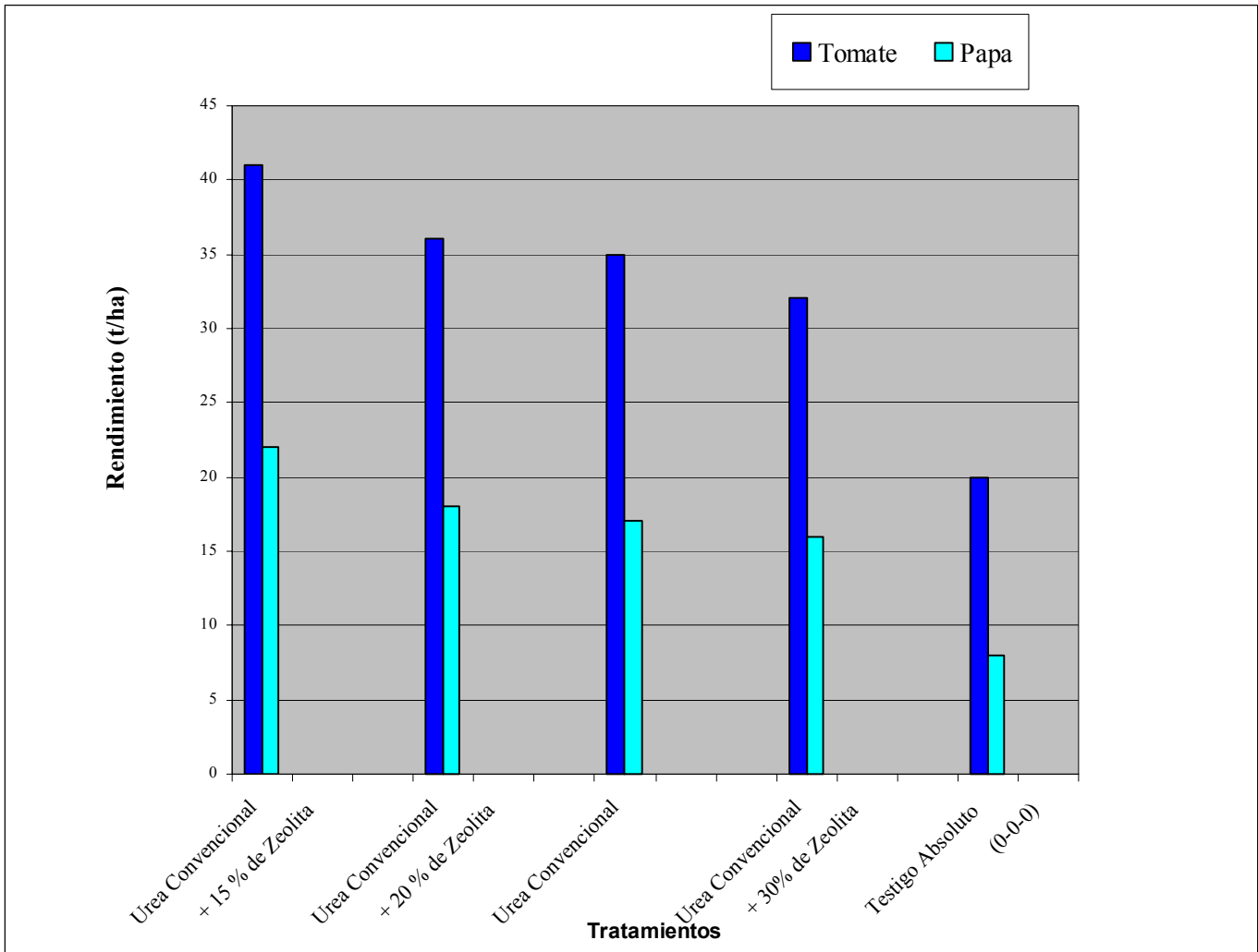
Graf. 1 Efecto de la urea mezclada con zeolita sobre los cultivos estudiados. Media de 3 años.
